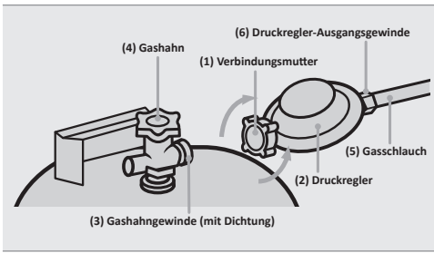
Abb.1: Montage des Druckreglers
