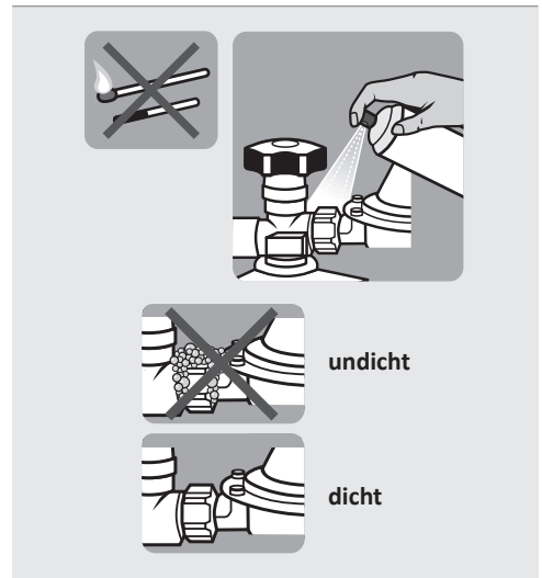
Abb.2: Dichtheitsprüfung
