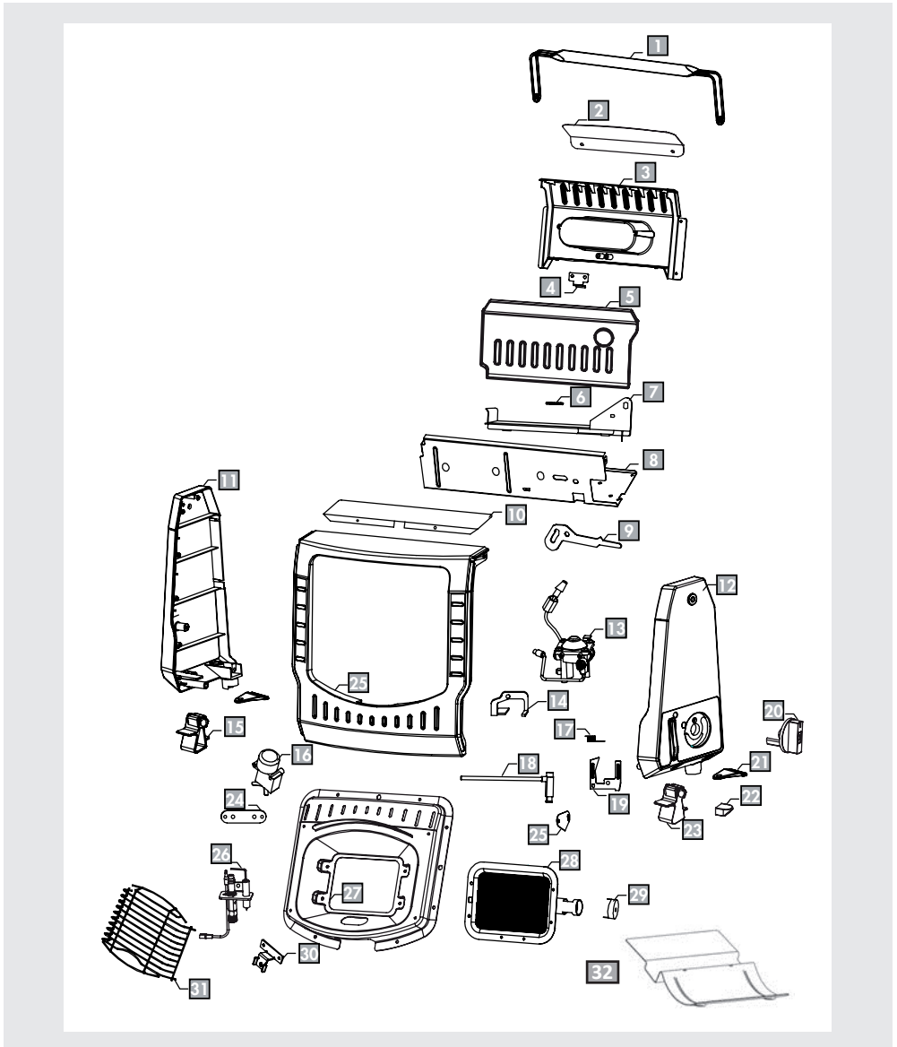
Abb. 4: Explosionszeichnung
